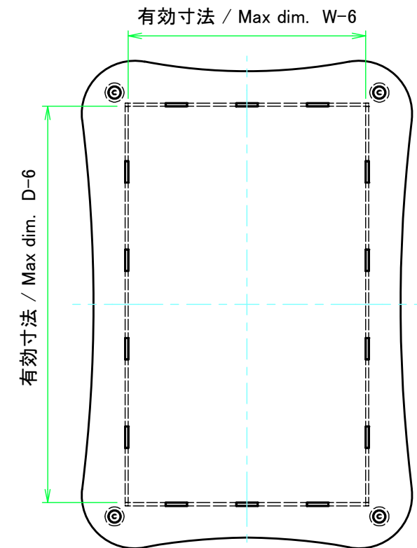
下カバー / Bottom cover
